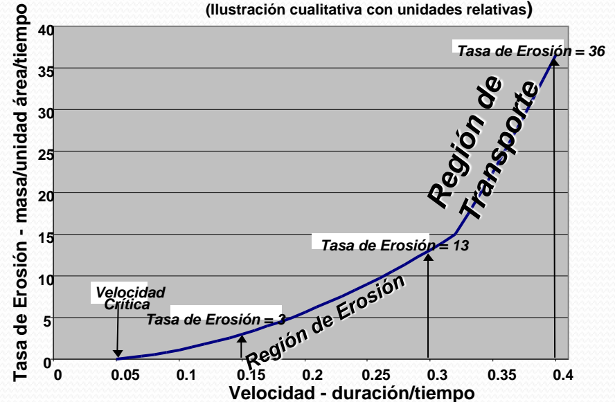
Efecto de la Velocidad en las Tasas de Erosión (Ilustración cualitativa con unidades relativas)
